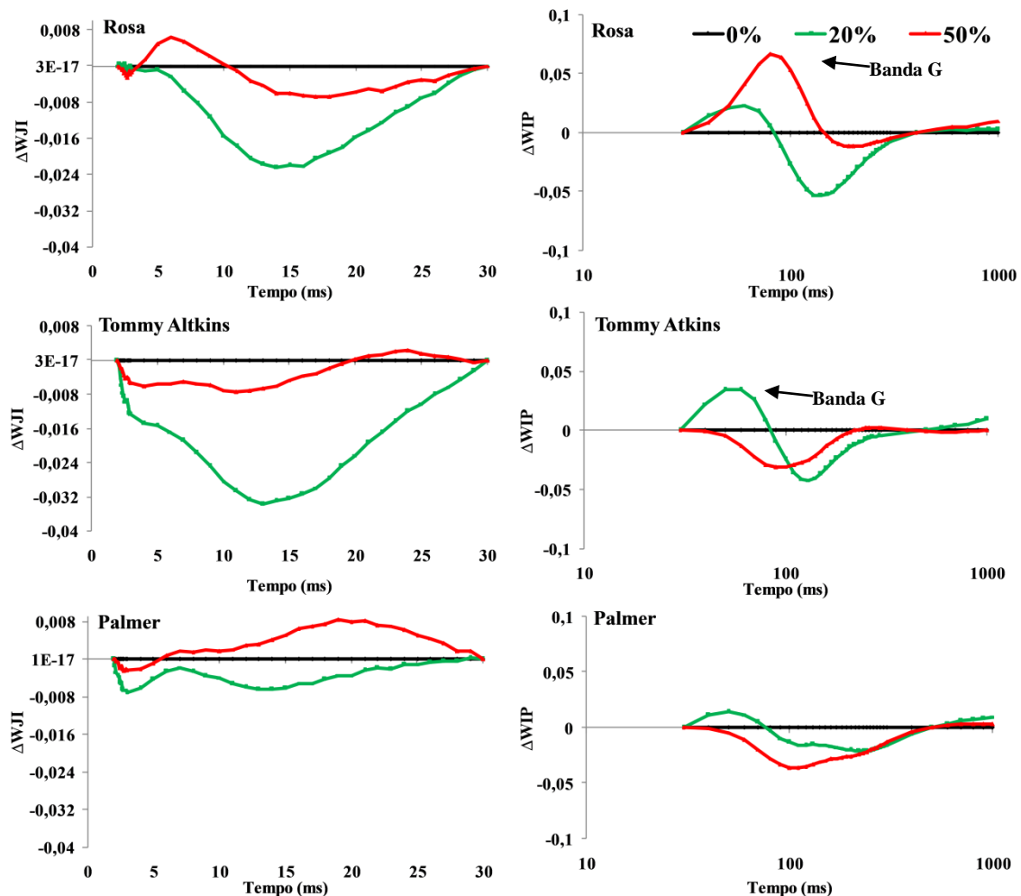
Figura 9: Diferenças cinéticas da fluorescência variável relativa entre as etapas J-I \Delta W_{JI} = (\Delta W_{JI(\text{tratamento})}) - (\Delta W_{JI(\text{controle})}) e I-P \Delta W_{IP} = (\Delta W_{IP(\text{tratamento})}) - (\Delta W_{IP(\text{controle})}) evidenciando o aparecimento da banda G. O tempo está representado em escala logarítmica (ms). (n=10)
