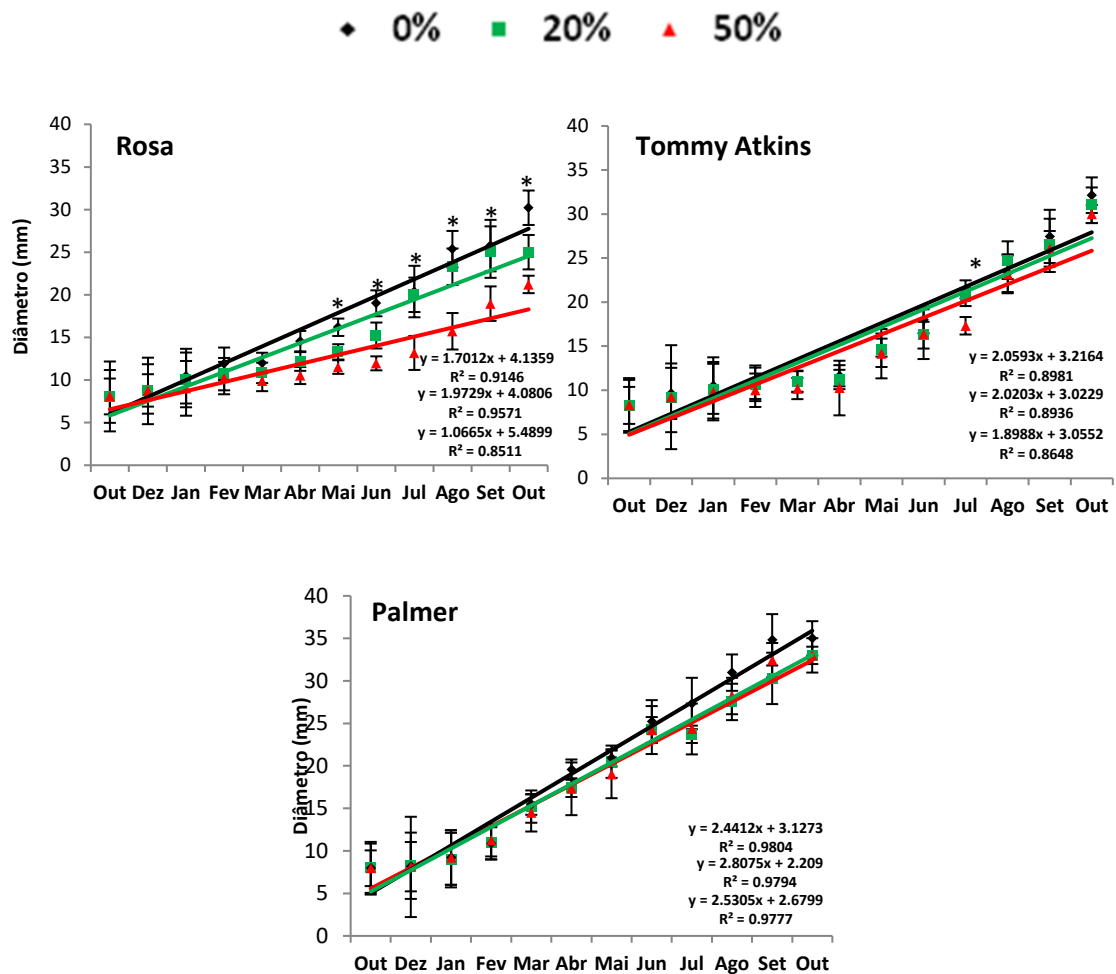
Figura 13: Diâmetro do caule ao longo dos meses desde estudo, de três cultivares de Mangifera indica L., cv.Rosa, cv.Tommy Atkins e cv.Palmer cultivadas em diferentes concentrações da lama, contendo resíduos de mineração, do Rio Doce.*Difere estatisticamente entre os tratamentos pelo teste Tukey ( \alpha=0.05 ). Barras representam o desvio padrão.(n=10)
