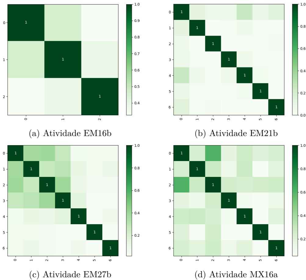
Figura 12 – Similaridade entre centroids para as atividades EM16b , EM21b , EM27b e MX16a em SciEntsBank .
