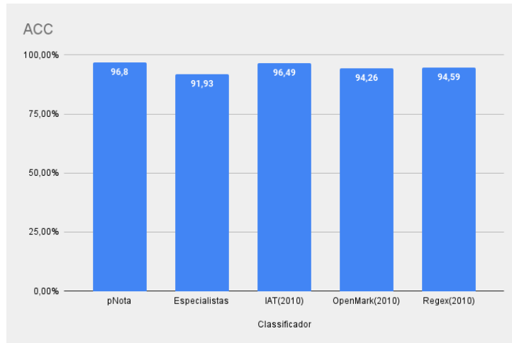
Figura 15 – Resultados obtidos no dataset Open University .
