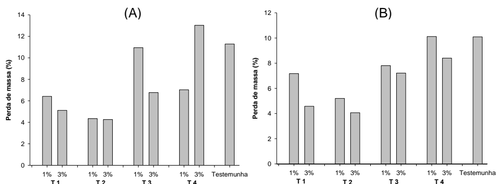
Figura 17. Perda de massa (%) no ataque de cupins em cada espécie, concentração (%) e tratamento: (A) B. vulgaris , (B) D. giganteus , (T1) transpiração diafragma íntegro, (T2) transpiração diafragma rompido, (T3) imersão prolongada, (T4) Boucherie modificado.
