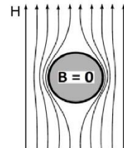
Efeito Meissner
