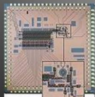
Microchip supercondutor Hypres com 6000 Junções Josephson
