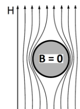
Fig. 1. Estado Supercondutor (Meissner) Seja - H: Campo Magnético Externo / B: Resposta Magnética do Supercondutor
