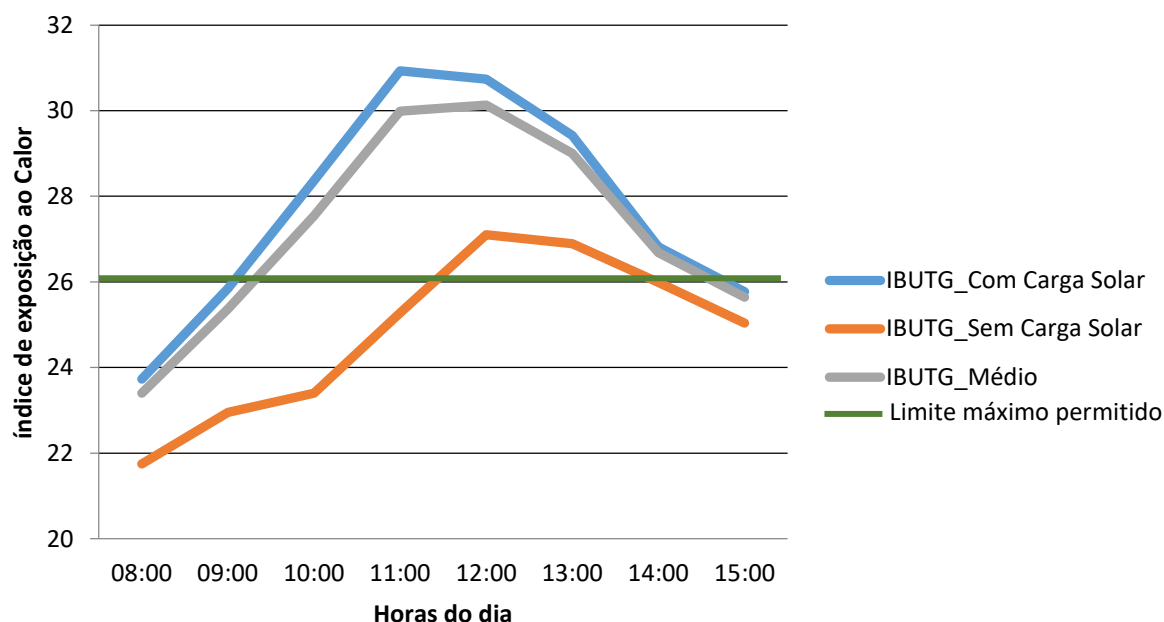
Figura 8 – Valores de IBUTG médios durante a jornada de trabalho
