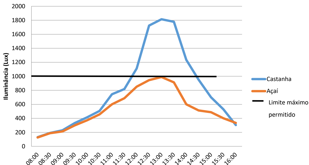
Figura 9 – Níveis médios de iluminância, em função do horário.
